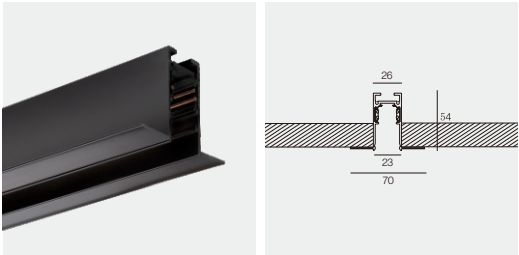
Mini Track M26T Trimless 095
