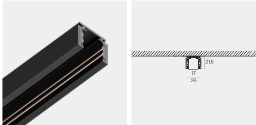
Mini Track M26S Surface 101
