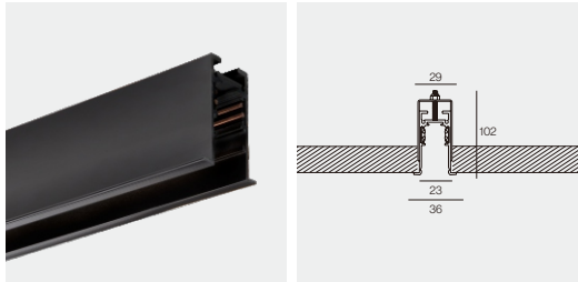
Mini Track M26R Trim 097
