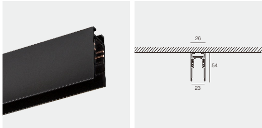
Mini Track M26A Suspended/Surface 093
