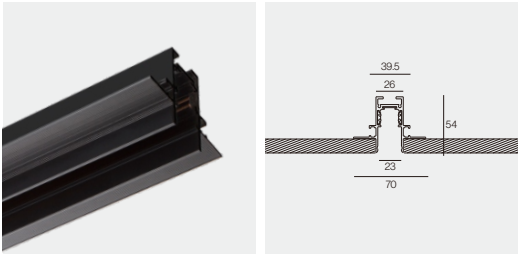
Mini Track M26E Trimless 099
