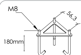
Art. 205 Kotwa do zabetonowania Art: 210, 211, 288, 289, 291, 293, 295, 296, 297, 298, 299, 1260, 1265, 1268, 1290, 1291, 1321, (1400- 1453) 1477, 1479, 1482, 1483, 1488, 1488
