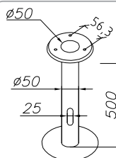
Art. 205 Kotwa do zabetonowania Art: 210, 211, 288, 289, 291, 293, 295, 296, 297, 298, 299, 1260, 1265, 1268, 1290, 1291, 1321, (1400- 1453) 1477, 1479, 1482, 1483, 1488, 1488
