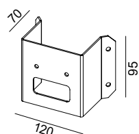
Art. 130 Narożnik Mandal Art: 1373, 1374
