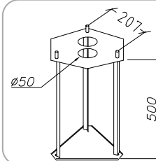
Art. 305 Kotwa do zabetonowania Art: 301, 302, 303, 382 Art: 362, 363, 364, 365 Art: 371, 372, 373 Art: 482, 483, 493, 492 Art: 810, 820, 830 Art: 951, 953
