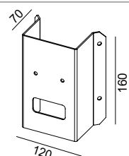
Art. 149 Narożnik Mandal Art: 1370, 1371
