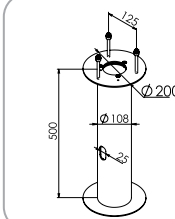
Art. 1230 Kotwa do zabetonowania Art: 1240, 1243, 1244, 1246, 1248, 1248 Art: 1280, 1285
