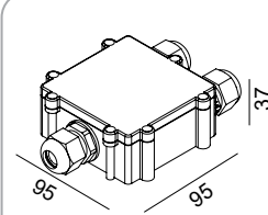
Art. 144 Puszka hermetyczna Egersund Mini, Lillesand, Oppland
