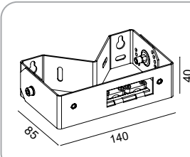
Art. 151 Narożnik z regulacją kąta świecenia Hitra
